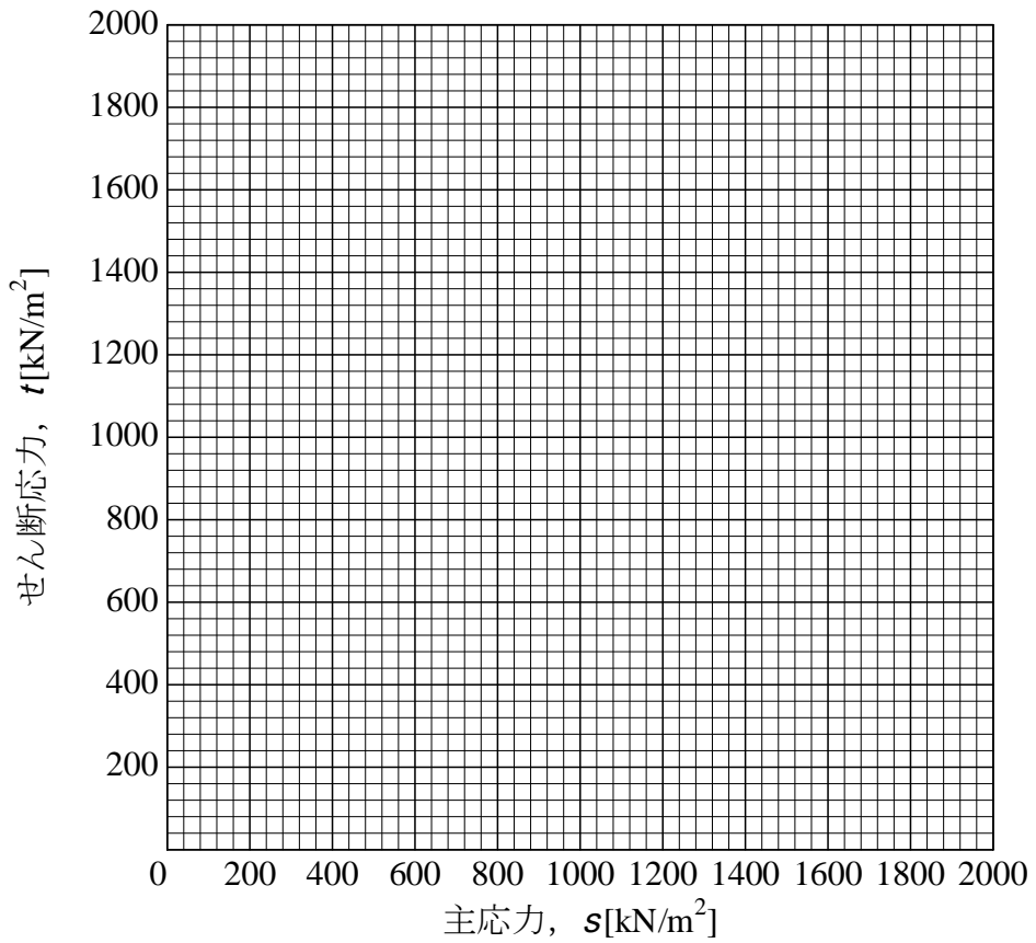
図-5 モール円 (非排水三軸圧縮試験) ※有効応力で整理すること
